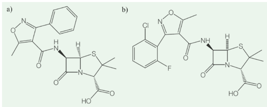
Obr. 1. Chemická struktura: a) oxacilinu; b) flukloxacilinu
